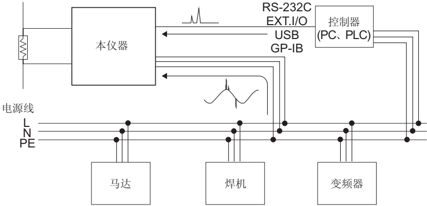
图.传导性噪音的进入
