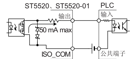
与PLC输入(负公共端子输入)的连接
