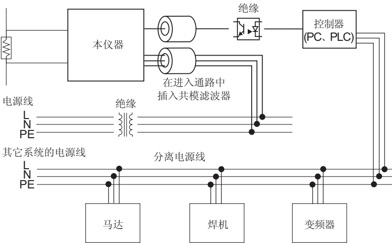
图.降低传导性噪音对策
