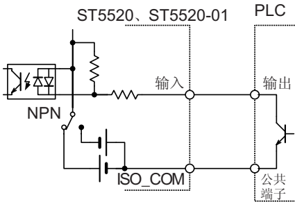
与PLC输出(NPN输出)的连接
