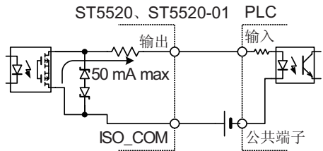
与PLC输入(负公共端子输入)的连接
