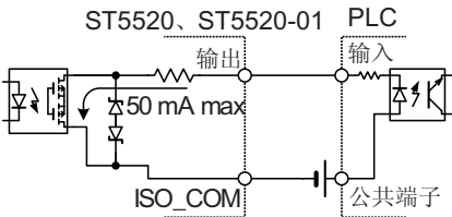
与PLC输入(正公共端子输入)的连接
