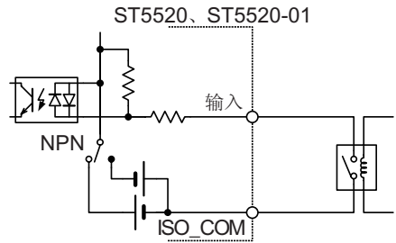
与继电器的连接
