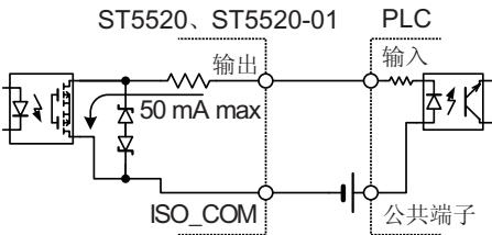
与PLC输入(正公共端子输入)的连接
