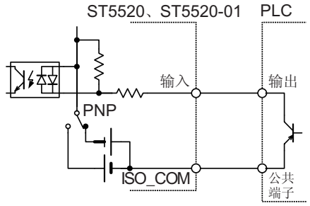
与PLC输出(PNP输出)的连接
