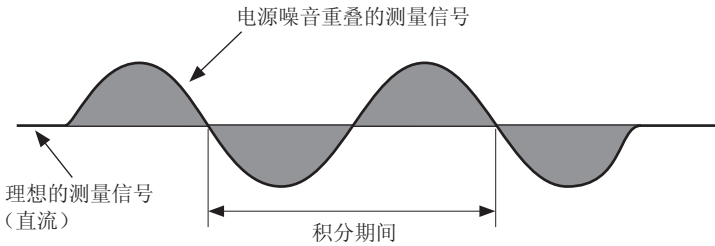
图.起因于工频电源的噪音
